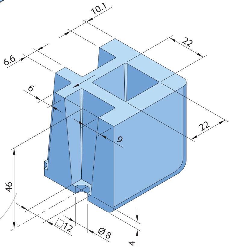
SECCIÓN ISOMÉTRICA
